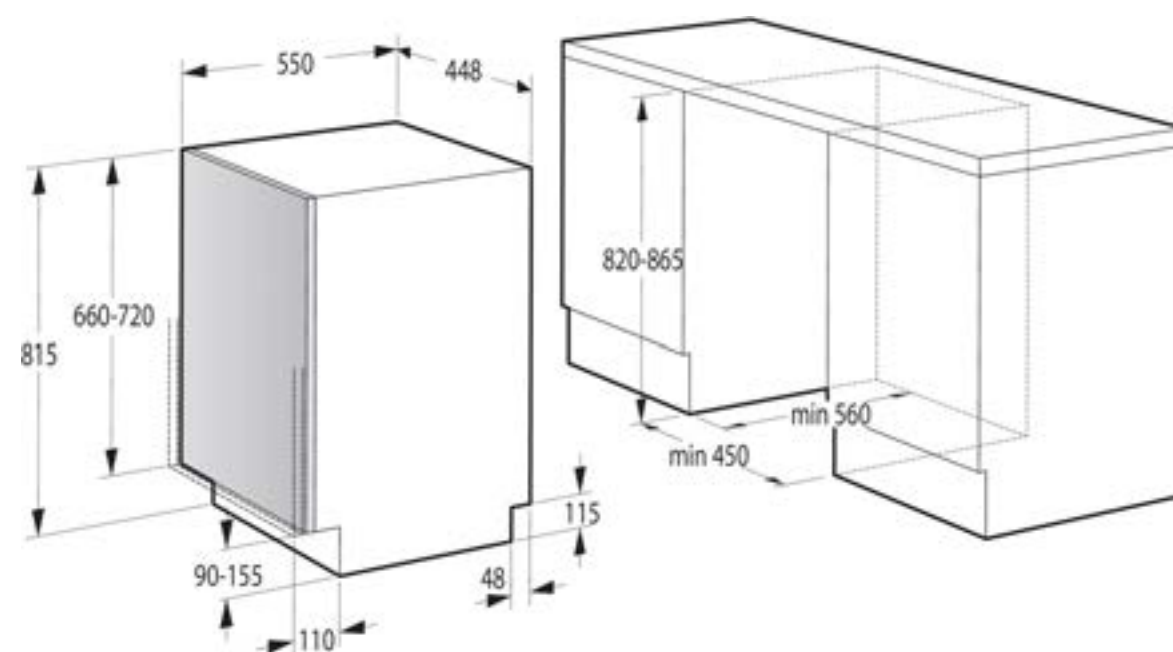
Disegno tecnico lavastoviglie slim HV523E10 _____
