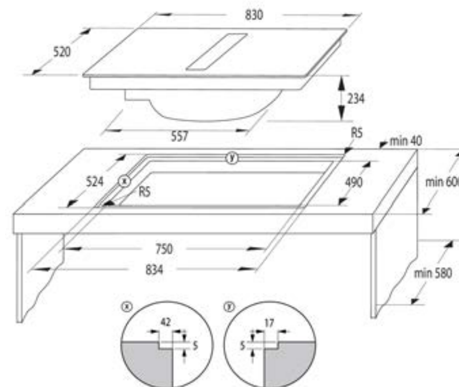
Piano cottura a induzione con cappa integrata da 80cm
