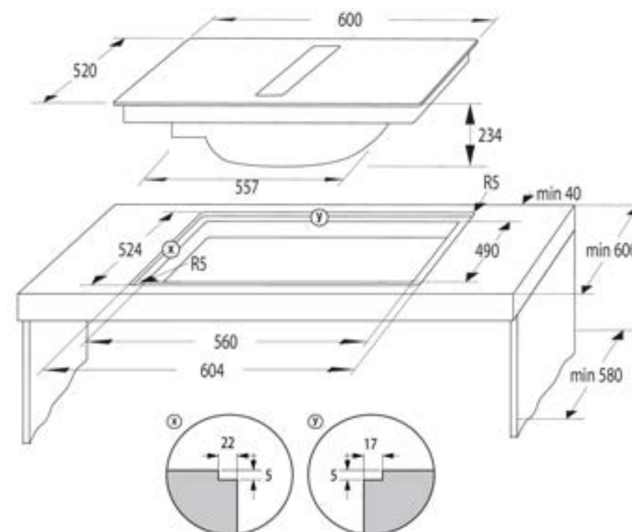
Piano cottura a induzione con cappa integrata da 60cm
