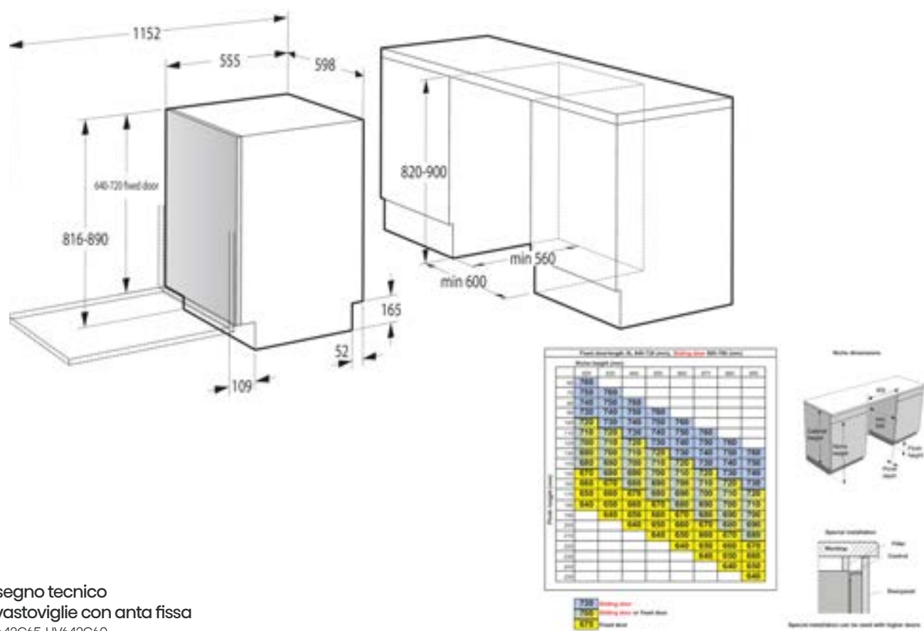
Disegno tecnico lavastoviglie con anta sliding HV693A65UVAD, HV673A65, HV693A62UVAD, HV673B61, HV673C61 HV663C62, HV643D62, HV642D62
