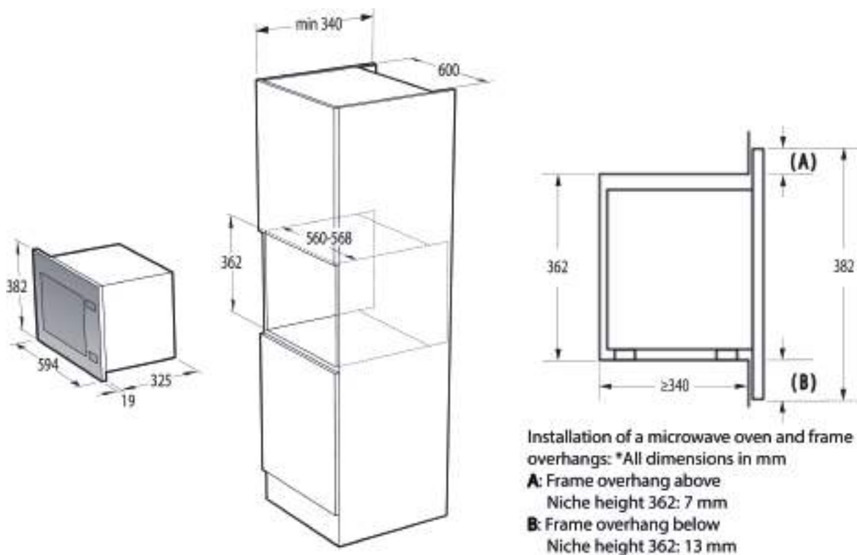
Disegno tecnico microonde a pensile
