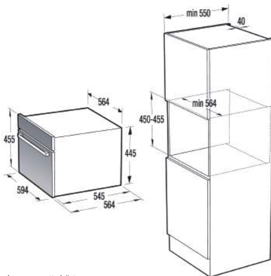
Disegno tecnico forno compatto full steam
