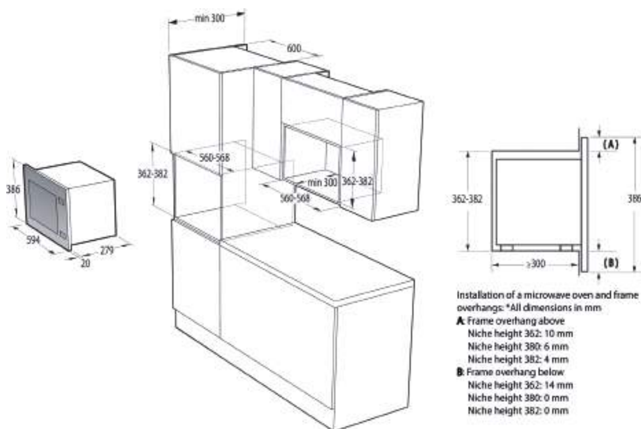
Disegno tecnico microonde
