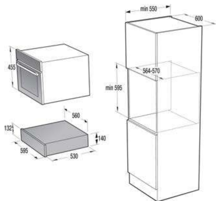
Disegno tecnico cassetto scaldavivande
