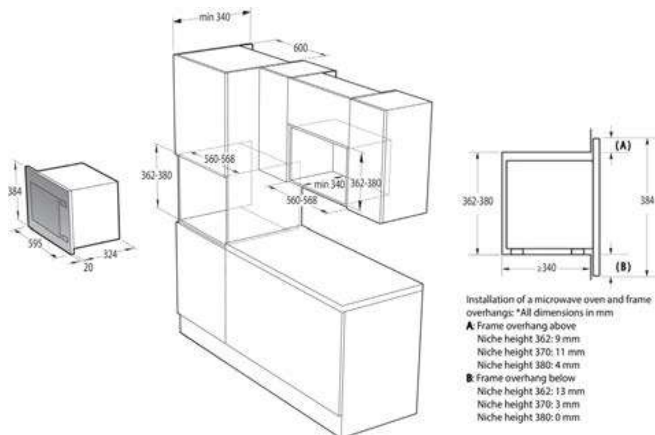
Disegno tecnico microonde a pensile
