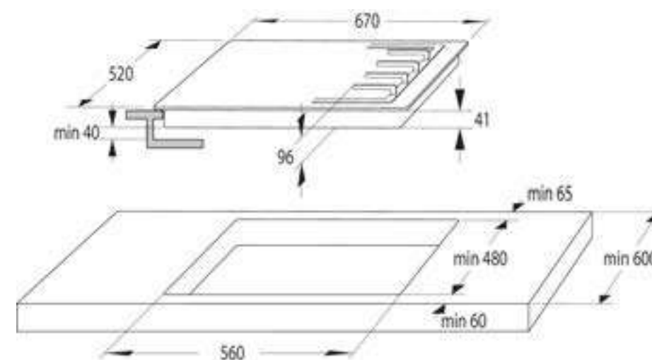
Disegno tecnico piani cottura a gas da 67cm GED663B, GMED663X
