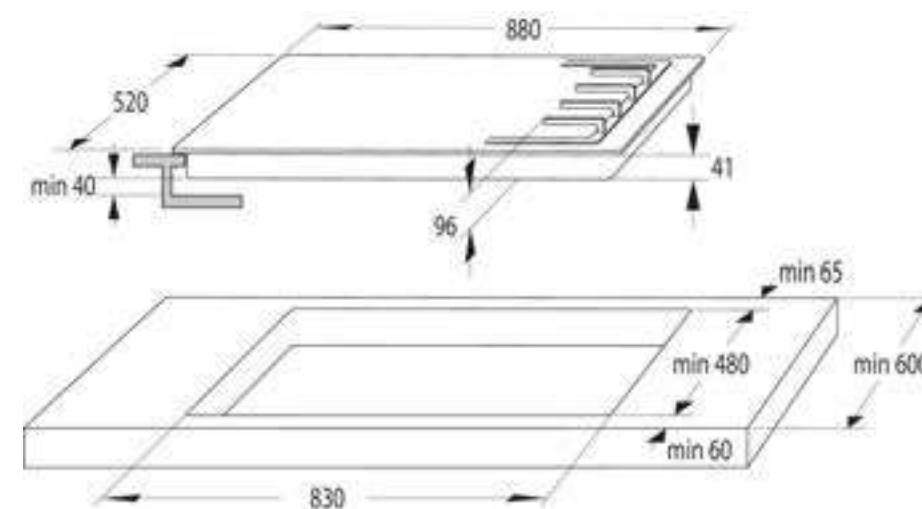
Disegno tecnico piani cottura a gas da 90cm GED973B, GMED973X
