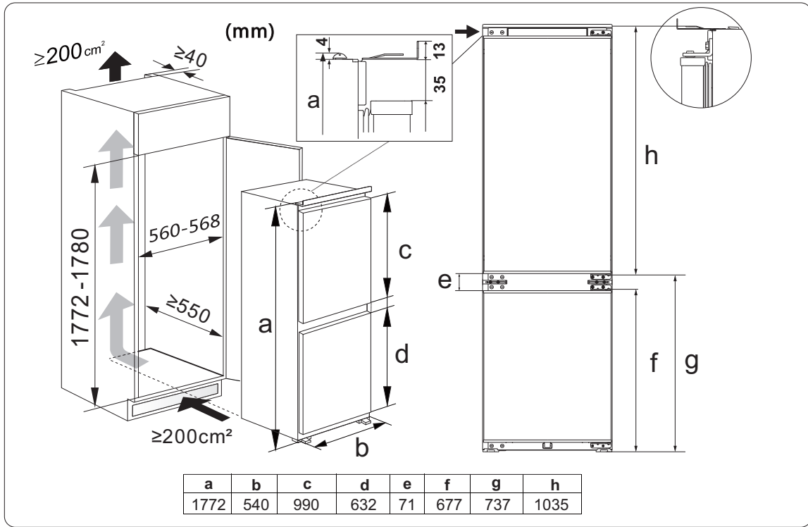
Disegno tecnico frigorifero RB3B280NEW1, RB3B250SAWE1
