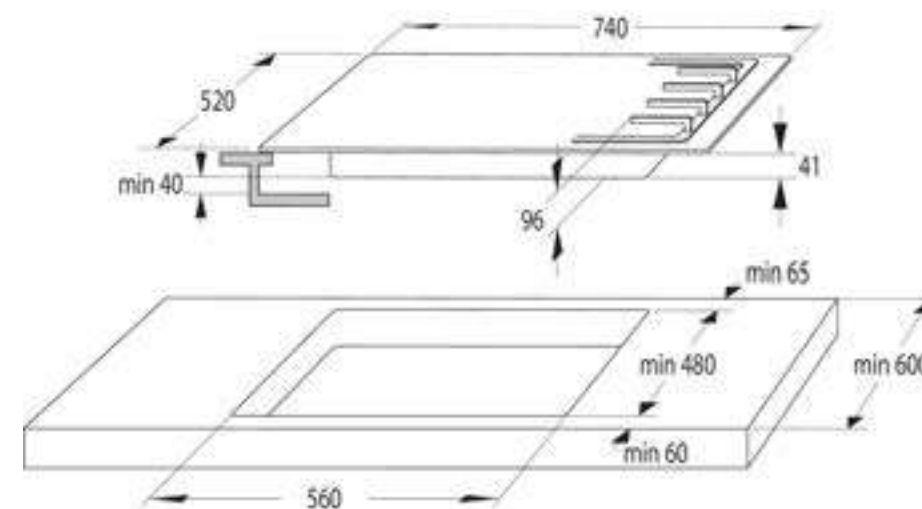
Disegno tecnico piani cottura a gas da 75cm GED773B, GMED773X
