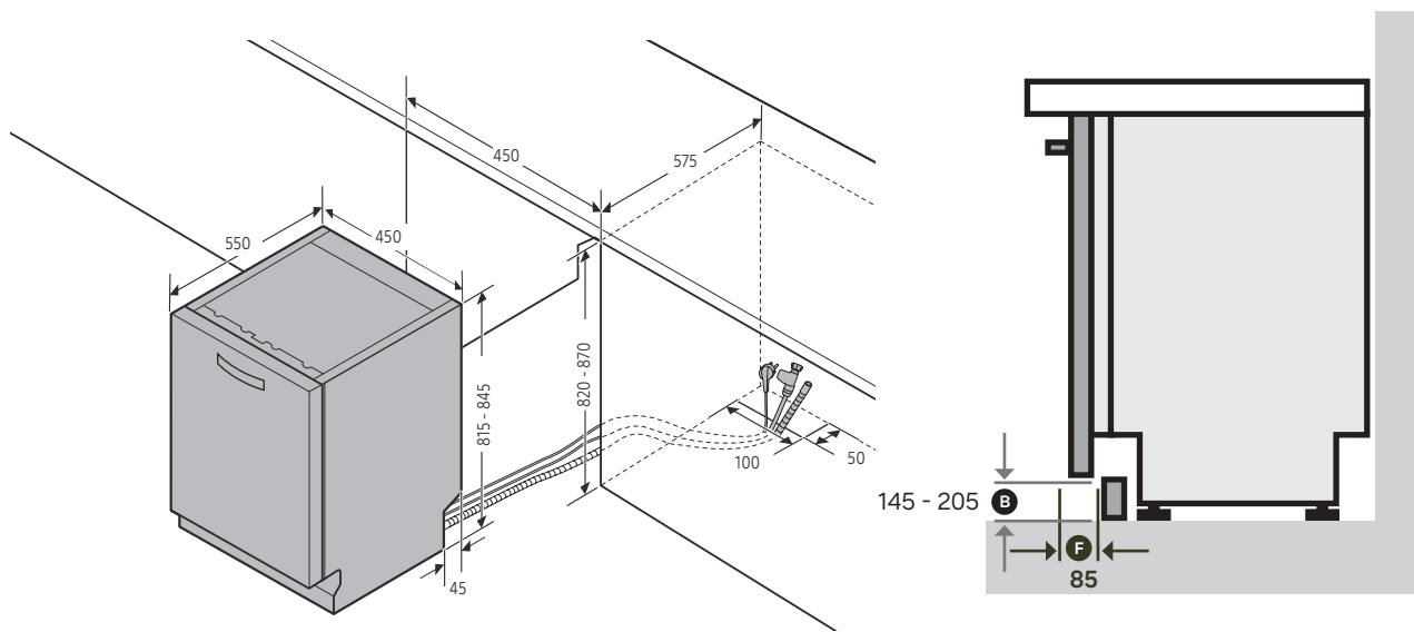
Dimensioni dell'armadiatura
