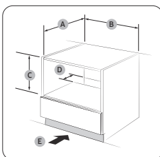
Struttura a incasso sotto lavello (mm)
