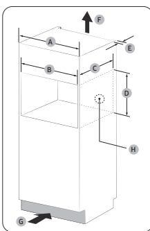
Struttura a incasso (mm)
