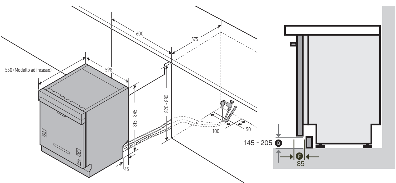
Dimensioni dell'armadiatura
