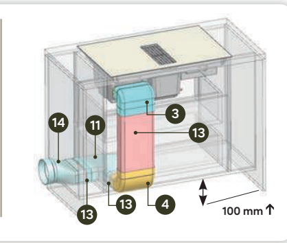
Kit Uscita Laterale (il kit rende possibile l'uscita sia a destra che a sinistra)
