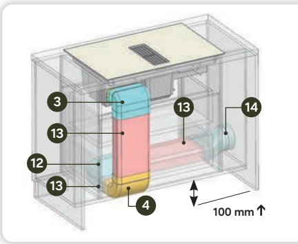
Kit Uscita Laterale (il kit rende possibile l'uscita sia a destra che a sinistra)
