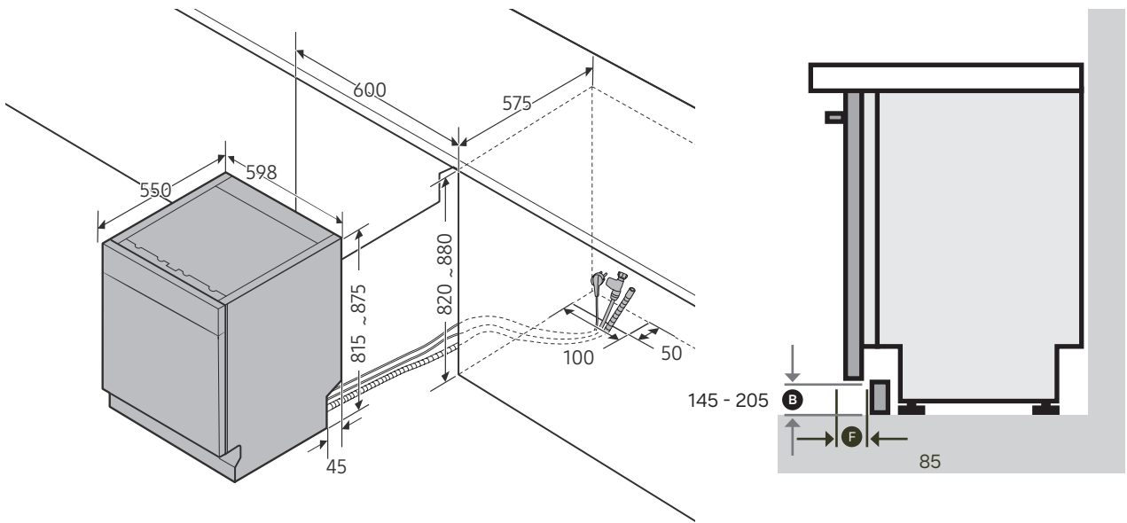
Dimensioni dell'armadiatura
