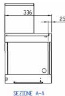
SEZIONE A-A
